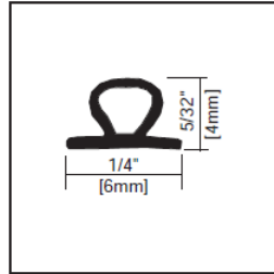
1/8" Gap Bulb w/Tape* VN.4057.CLR - SDTJ
