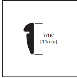
3/8" Panel Glazing Vinyl VN.4033.CLR (Use EX.1018)
