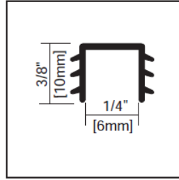
1/4" Hdr Glazing Vinyl VN.4001.CLR (Use EX.1587)
