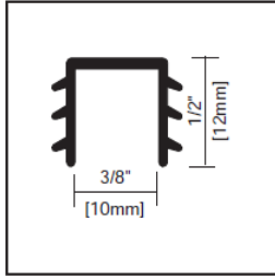
3/8" Hdr Glazing Vinyl VN.4010.CLR (Use EX.1082)
